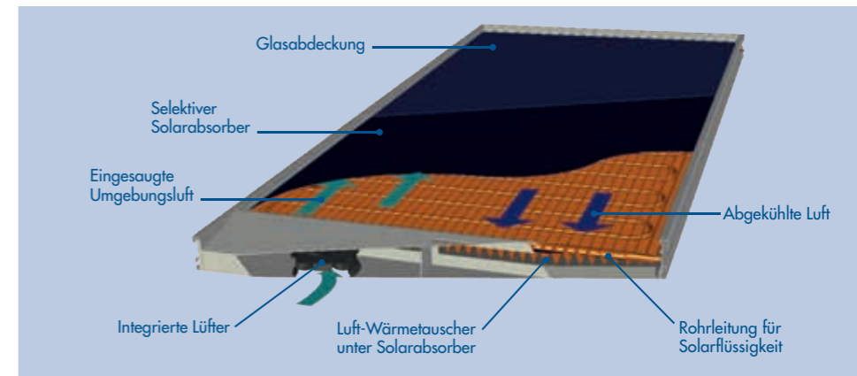
Querschnitt durch den patentierten Hybridkollektor, der auf 2 unterschiedliche Arten Wärme gewinnen kann.
